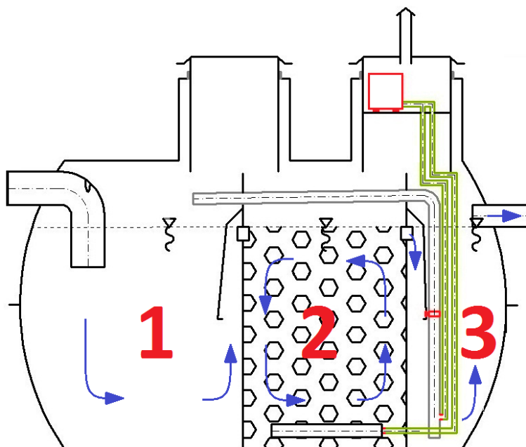
1. Osadnik wstępny (OWS), 2. Reaktor biologiczny (RB), 3. Osadnik wtórny (OWT)
