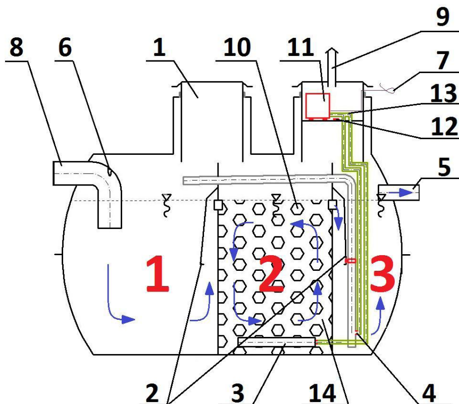
Schemat 2. Opis techniczny przydomowej oczyszczalni ścieków BIO-HYBRYDA
